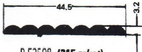
B-E2508 (315 gr/mt)
