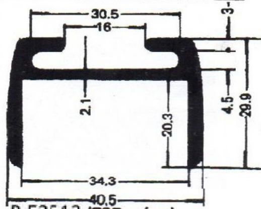
B-E2513 (785 gr/mt)
