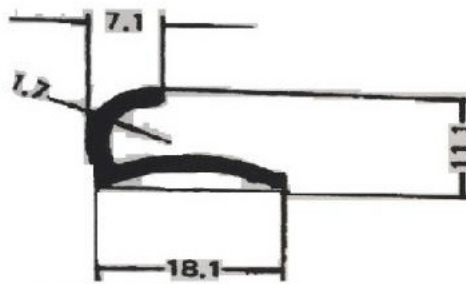
B-E2524 (125 gr/mt)
