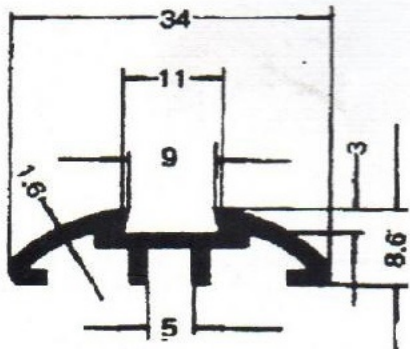
B-E2510 (290 gr/mt)
